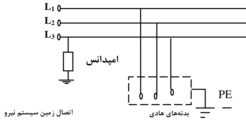
شکل پ ۵ سیستم TT
